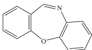
dibenzo[b,f][1,4]oxazepine
